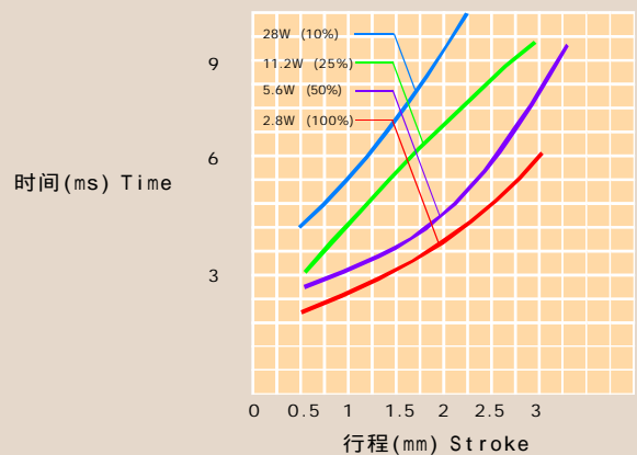
行程/响应时间 Stroke and Time
