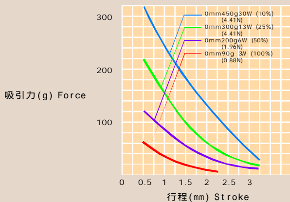
行程/吸引力 Stroke and Force
